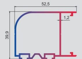
T.2156 0,650 kg/mt Köşe Dönüş Profili
