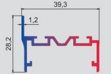
T.2155 0,374 kg/mt Ara Fital Profili
