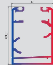
T.2151 1,580 kg/mt Kasa Profili
