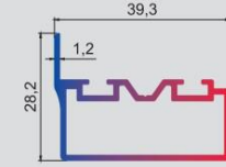
T.2154 0,463 kg/mt Yan Dikme Profili
