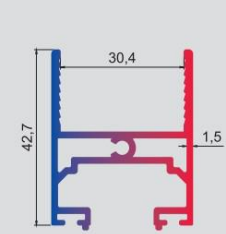
T.2153 0,800 kg/mt Kanat Profili
