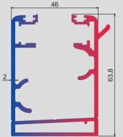
T.2152 1,629 kg/mt Damlalık Kasa Profili
